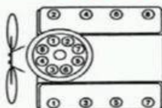
CHRYSLER CORP. V-8 383-440 CID (BIG BLOCK)
