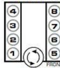
FORD 5.0L EFI 351W, 351, 400
