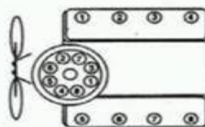
FORD MOTOR CO. V-8 351W, 351C, 351M, 400M CID
